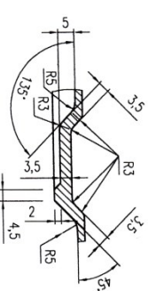
CHI TIẾT III TL 5:1
