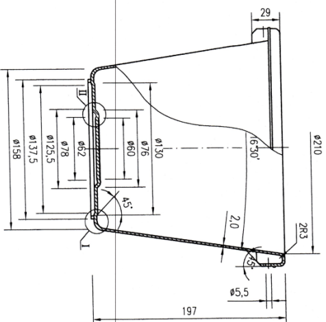
MẶT CẮT ĐÚNG 1
