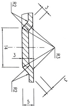
CHI TIẾT II TL 5:1
