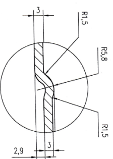
CHI TIẾT II
