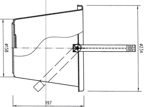
MẶT ĐÚNG 2
