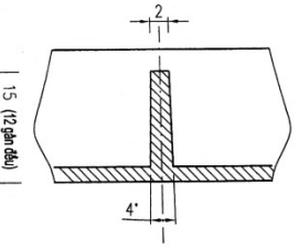
MẶT CẮT A-A TL 4:1
